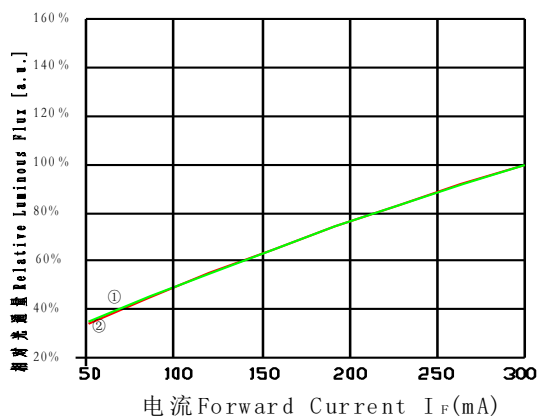
Forward Current vs. Relative Luminous Flux 正向电流与相对光通量曲线图
