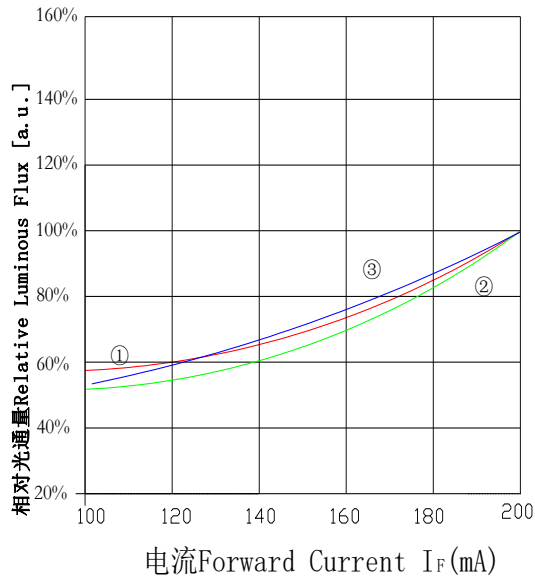
Forward Current vs. Relative Luminous Flux 正向电流与相对光通量曲线图
