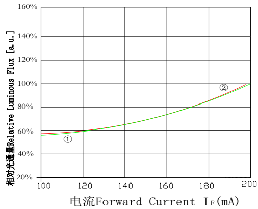
Forward Current vs.Relative Luminous Flux 正向电流与相对光通量曲线图
