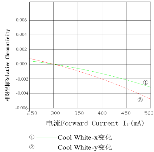
Cool White Current vs. Relative Chromaticity 冷白电流与相对坐标变化曲线图
