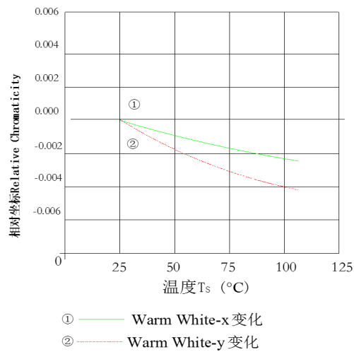
Warm White Temperature vs. Relative Chromaticity ( I_F=500\text{mA} ) 暖白线路温度与相对坐标变化曲线图
