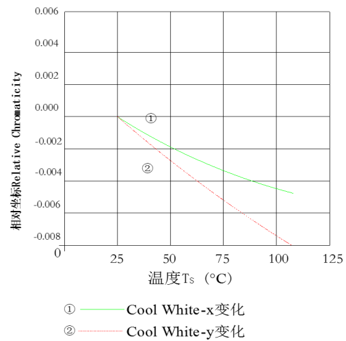
Cool White Temperature vs. Relative Chromaticity ( I_F=500\text{mA} ) 正白线路温度与相对坐标变化曲线图
