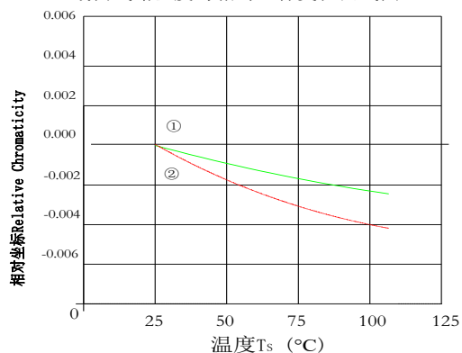
Warm White Temperature vs. Relative Chromaticity (IF=250mA) 暖白线路温度与相对坐标变化曲线图
