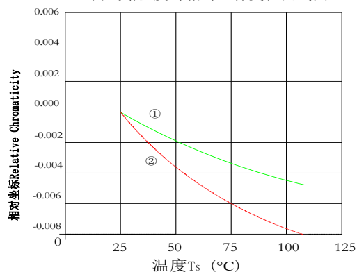
Cool White Temperature vs. Relative Chromaticity (IF=250mA) 正白线路温度与相对坐标变化曲线图
