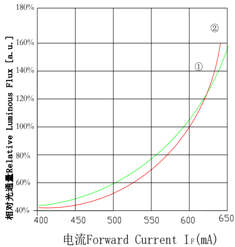
Forward Current vs. Relative Luminous Flux 正向电流与相对光通量曲线图
