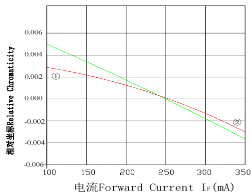
Cool White Current vs. Relative Chromaticity 冷白电流与相对坐标变化曲线图
